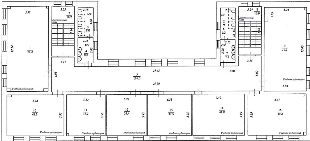
План 4 этажа
