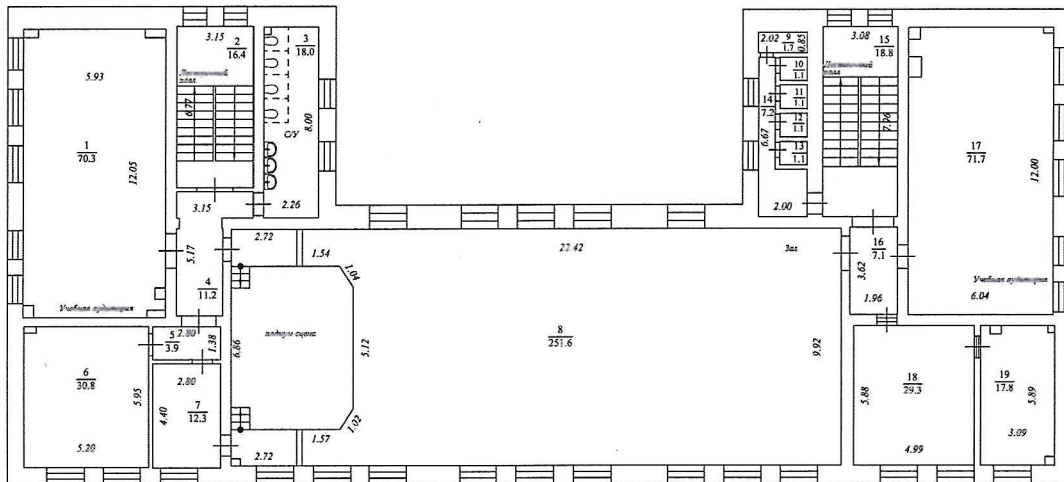
План 5 этажа
