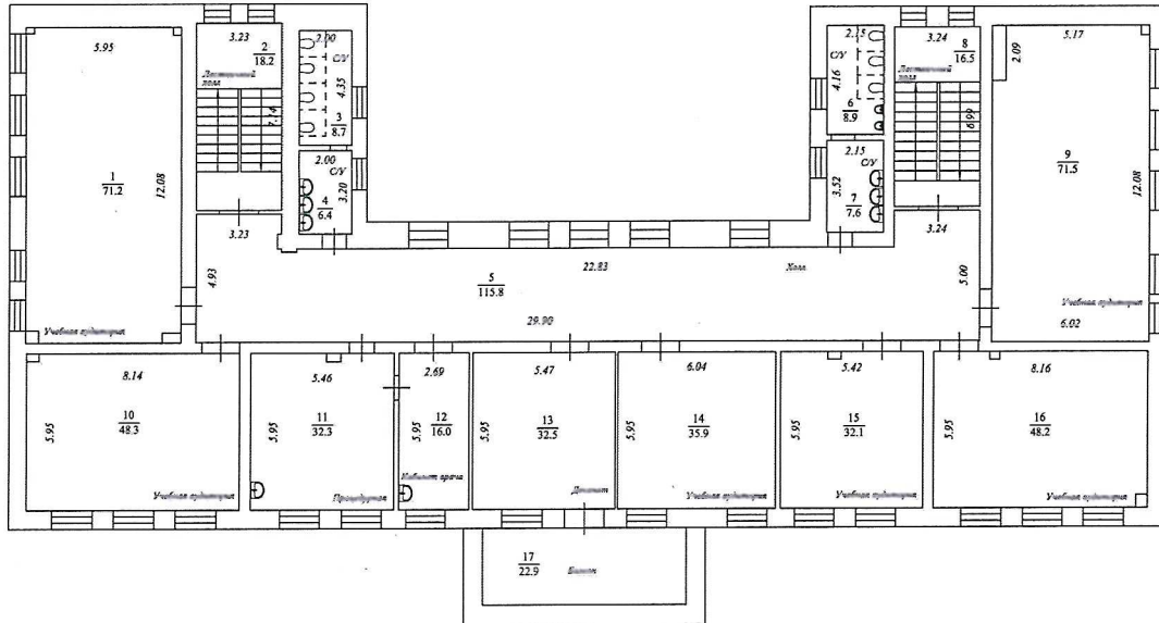
План 2 этажа
